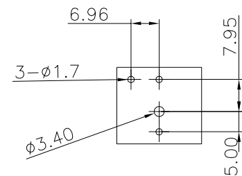
P.C.B Layout (1:1)
