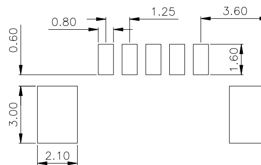
P.C.B Hole Layout
