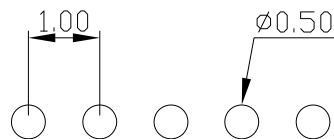
P.C.B Hold Layout
