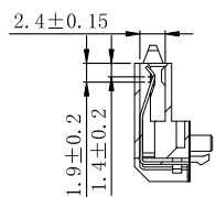
剖視圖 A-A
